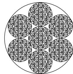
Konstruktion 6x19
