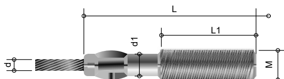
Gewindebolzen zum Verpressen
