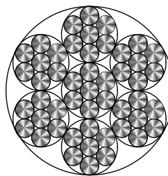
Konstruktion 7x7
