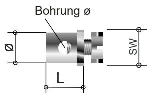
Schraubnippel mit Schlüsselansatz, Sechskantschraube
