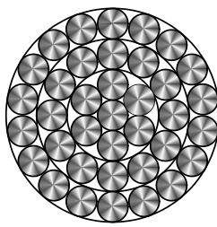
Konstruktion 1x37
