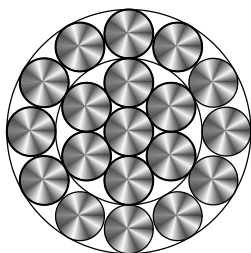
Konstruktion 1x19
