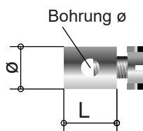
Schraubnippel mit Sechskantschraube und Schlitz
